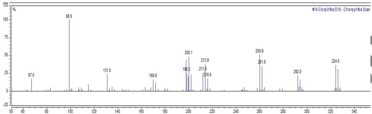
Figura 2. Espectro de masas Clorpirifos (D10)
