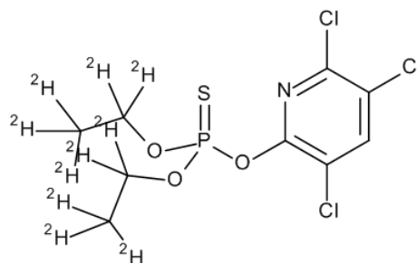
Figura 1. Estructura molecular del Clorpirifos (D10)
